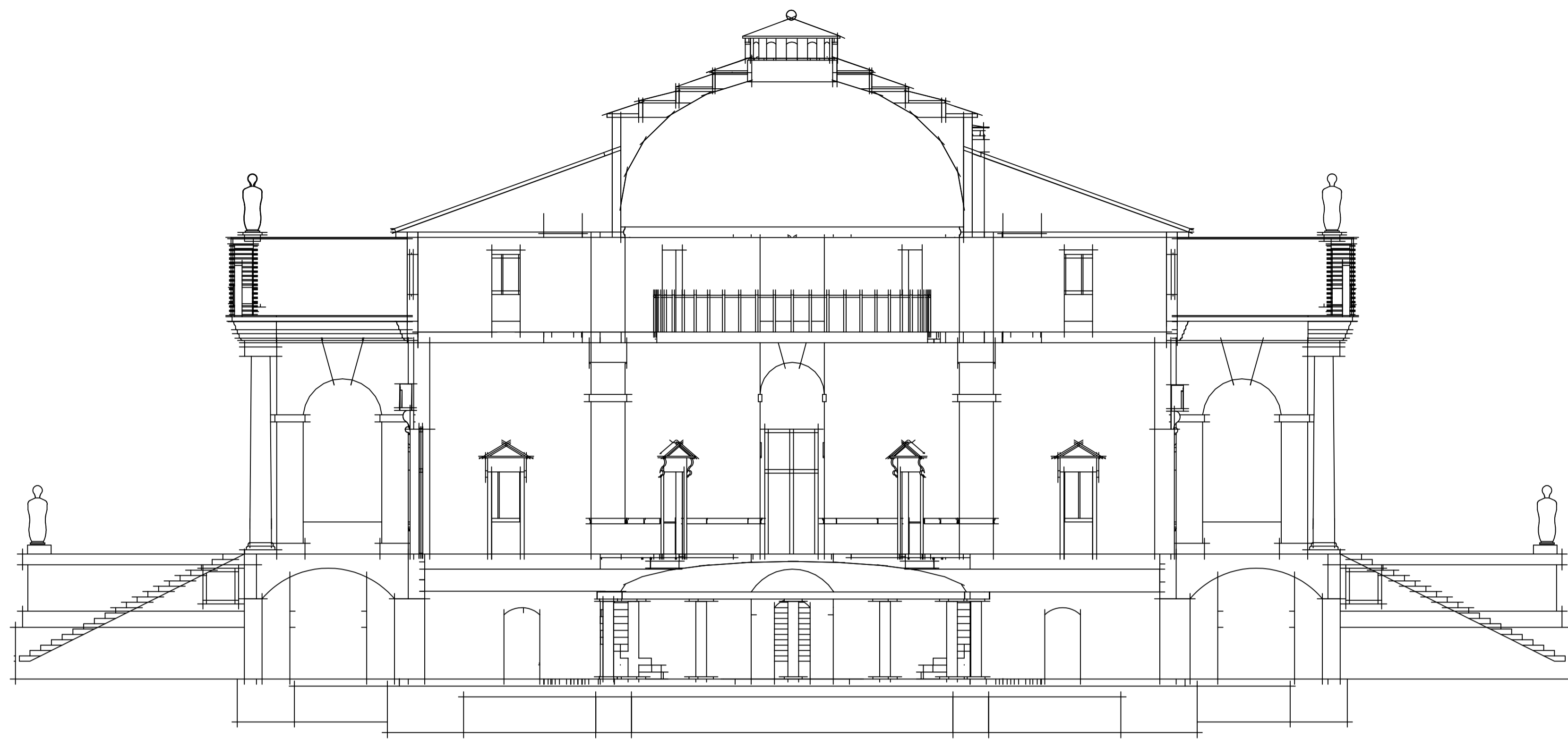
CORTE
