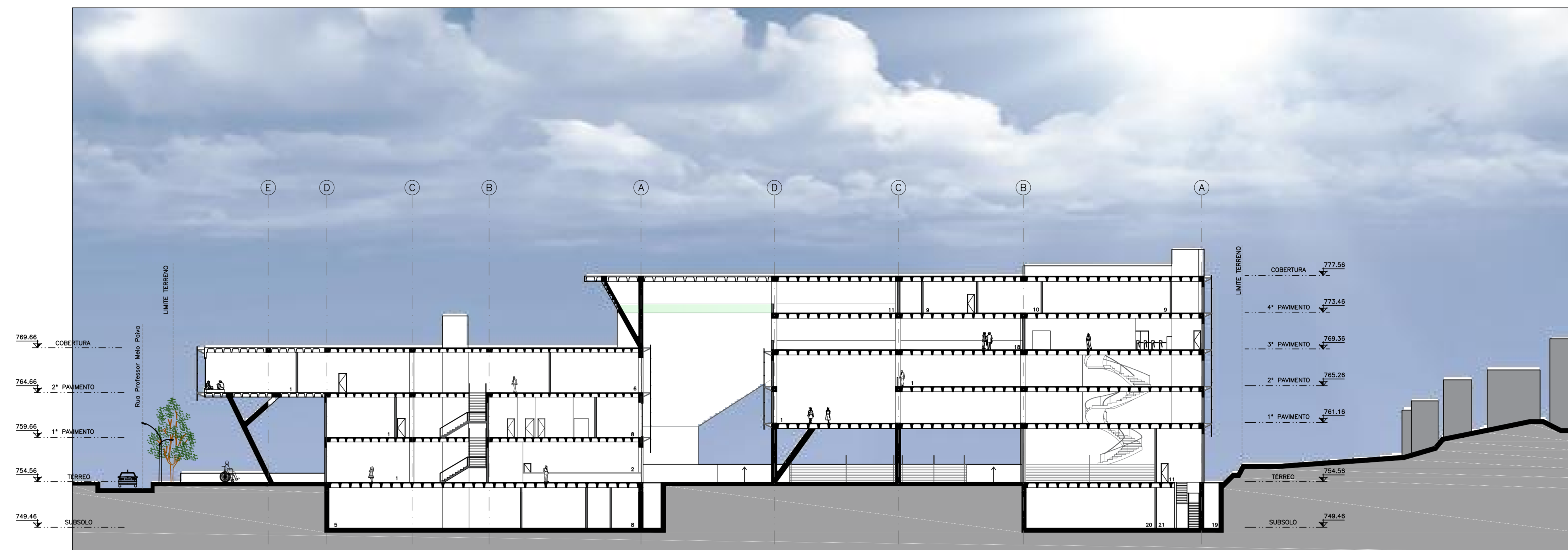
CORTE BB esc. 1:300
