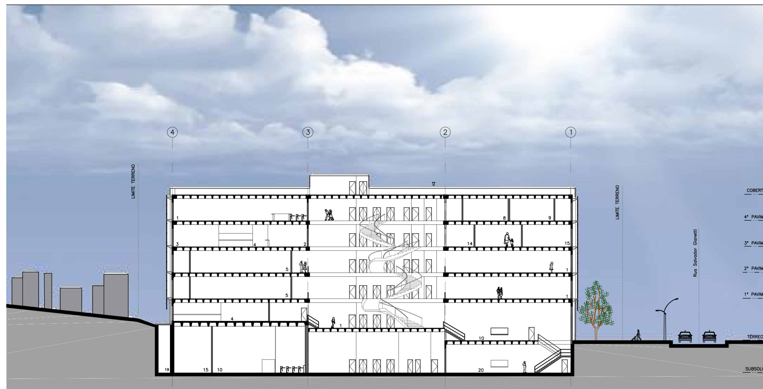
CORTE AA esc. 1:300
