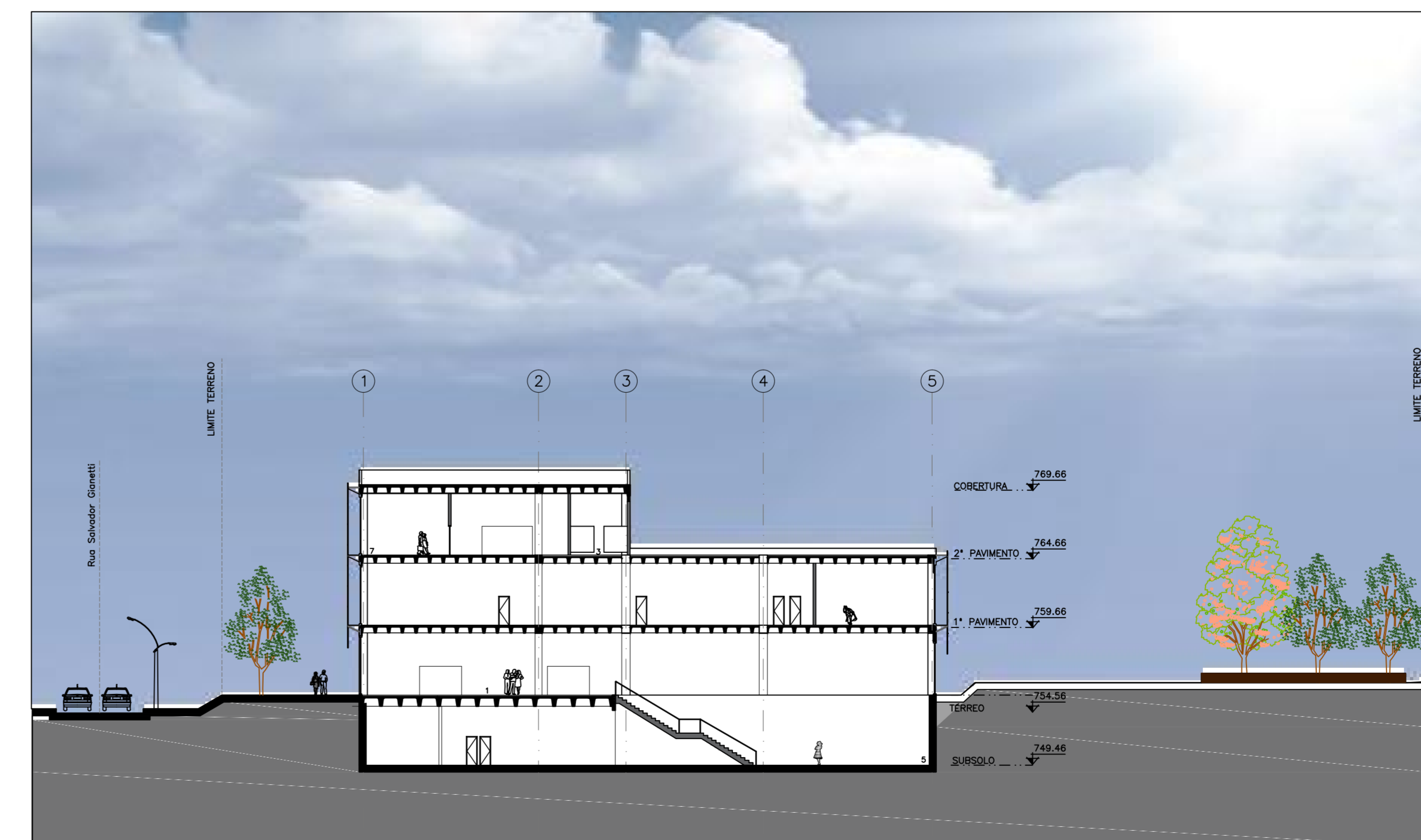
CORTE DD esc. 1:300
