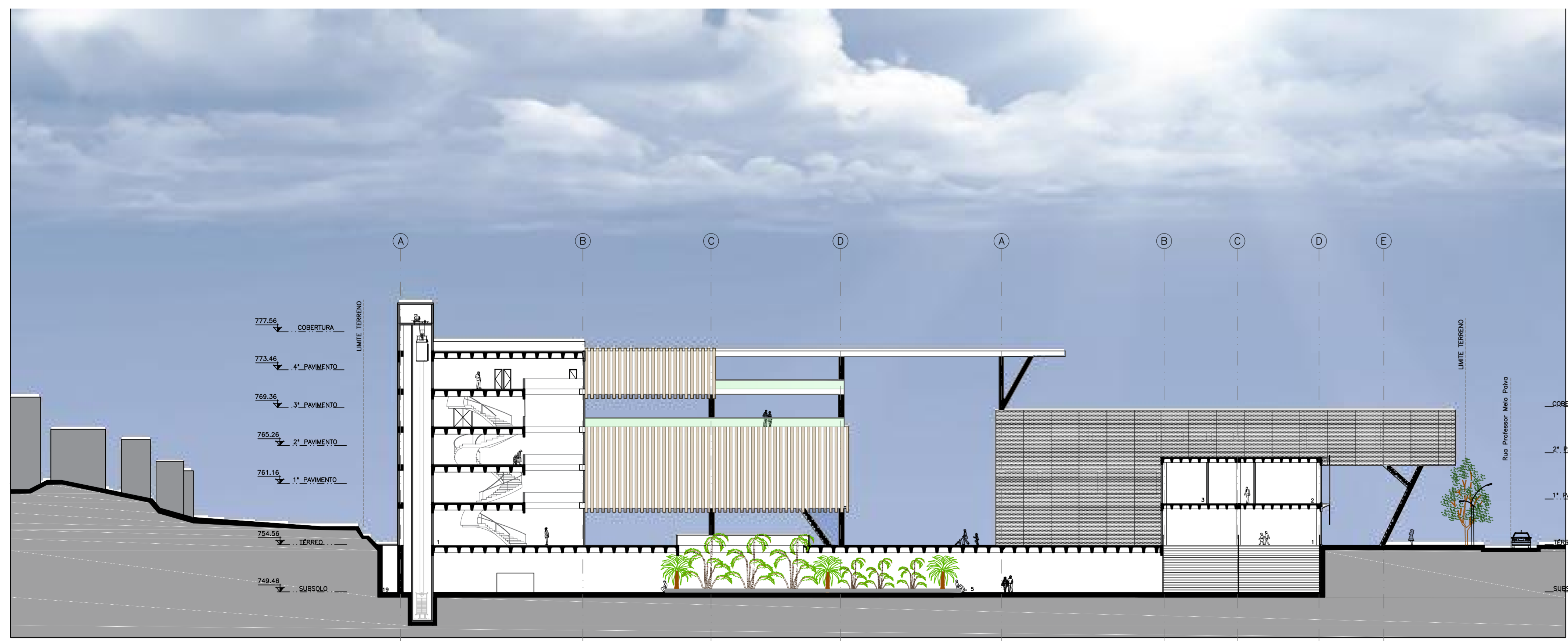
CORTE CC esc. 1:300
