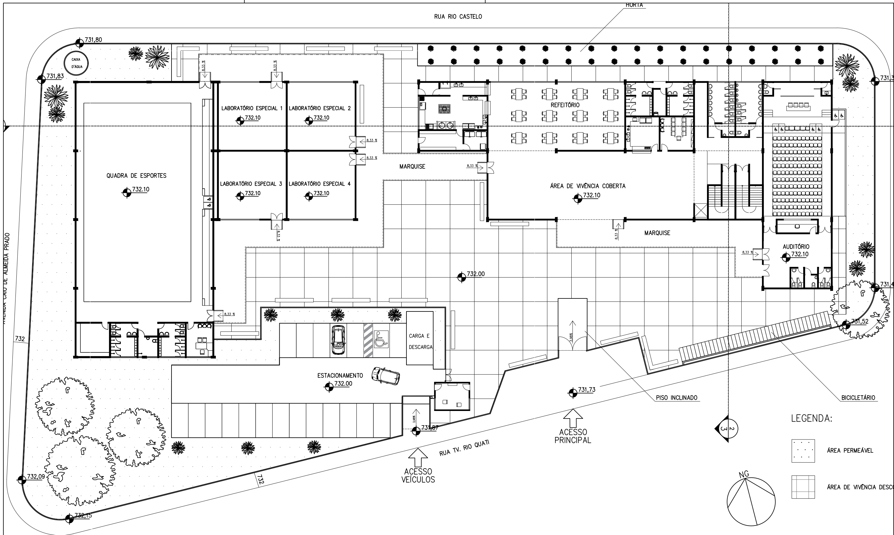
1 PLANTA PAVIMENTO TÉRREO ESCALA 1:300
