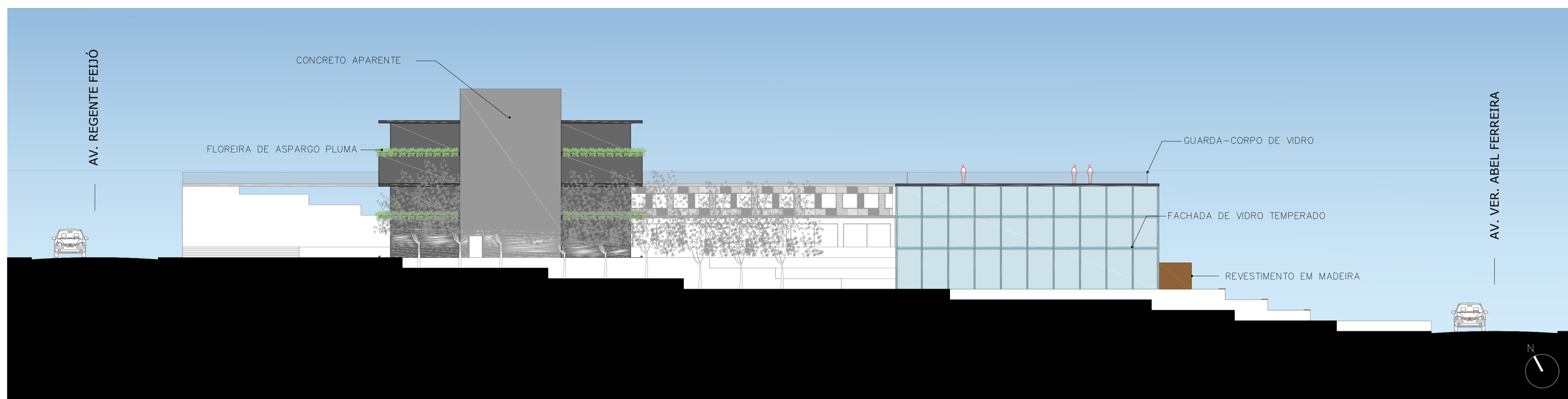
FACHADA 3 - BLOCO 1 E BLOCO 4 ESCALA 1/250
