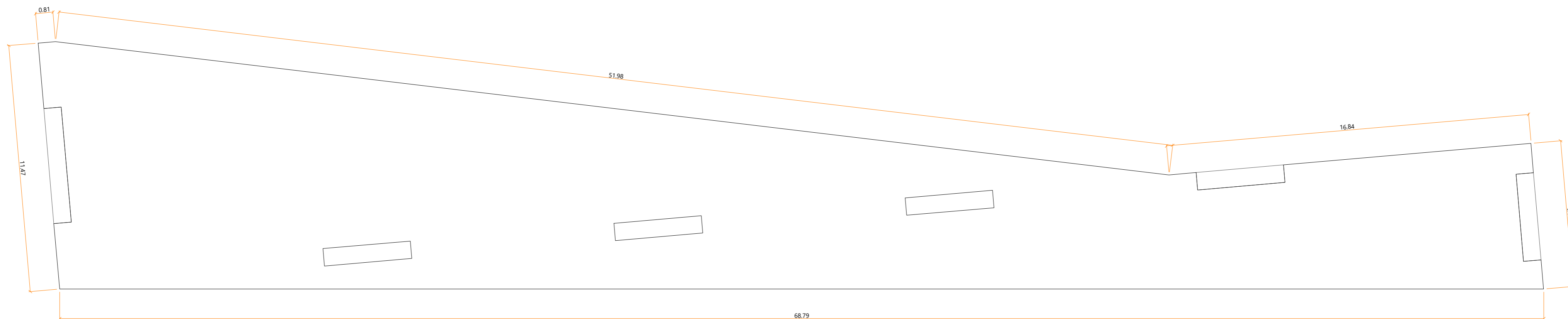
VISTA LATERAL CAIXA PORTA REGISTRO - FOLHETARIA / CCSP MDF 6MM esc 1/1
