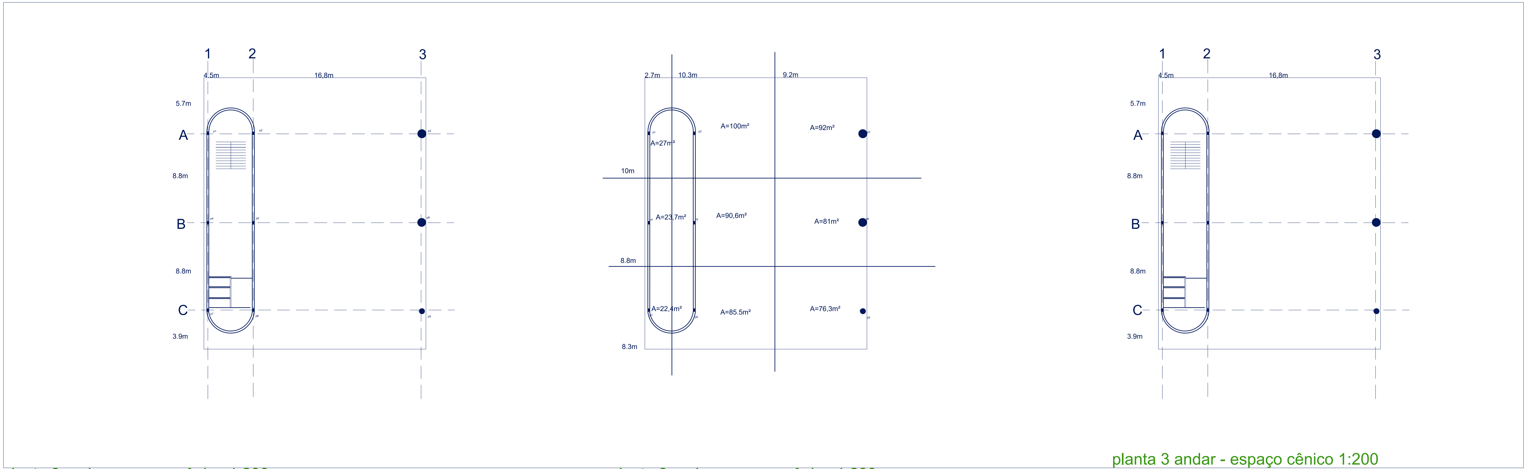
planta 3 andar - espaço cênico 1:200
