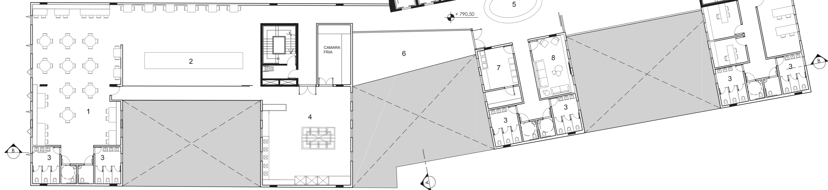
SERVIÇOS E ADMINISTRATIVO - 3º PAVIMENTO ESCALA: 1/300
